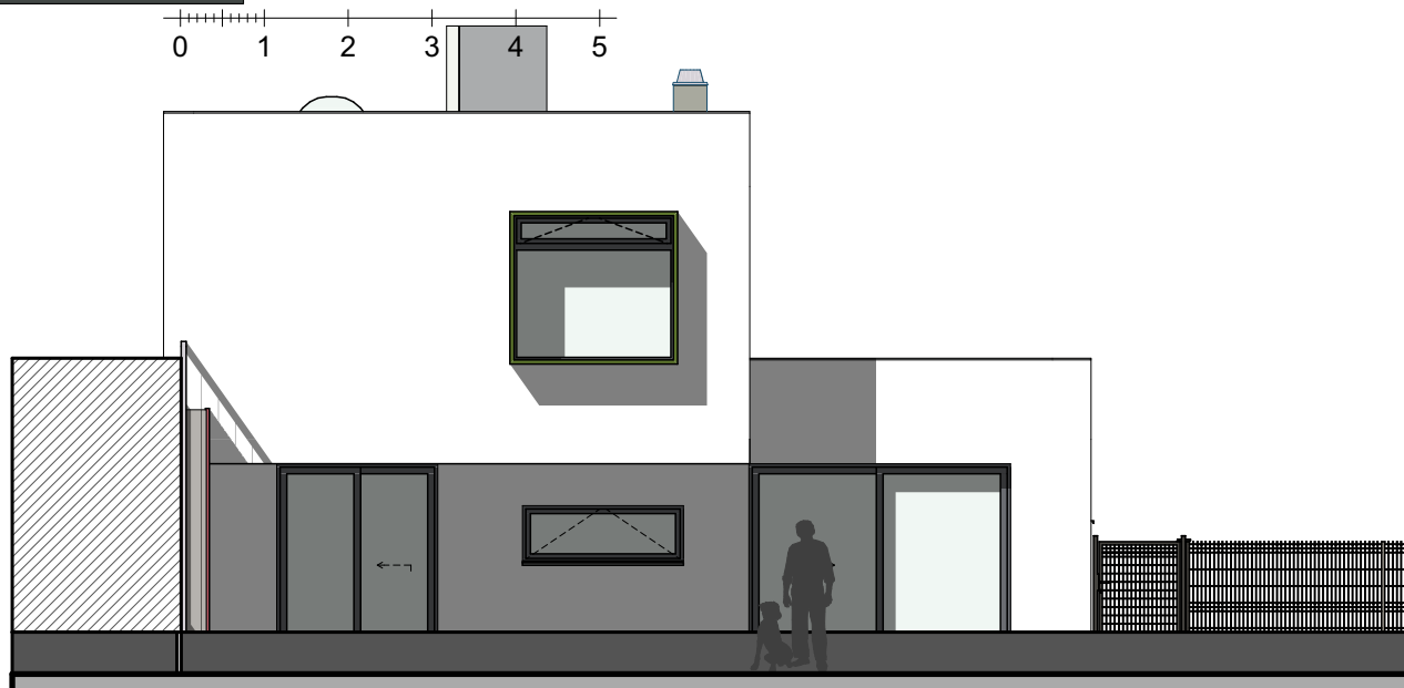
Pohled Západní
